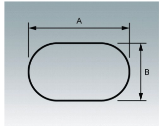
M0000801 Ausschnitt, oval Stanzwerkzeuge
