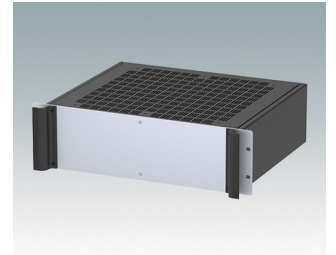
M6219369 COMBIMET 19" 3HEx365mm Mit Lüftung Aluminium Schwarz RAL 9005 132.5x482.6x365mm
