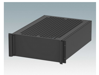
M6219489 COMBIMET 19" 4HEx610mm Mit Lüftung Aluminium Schwarz RAL 9005 177x482.6x609.6mm
